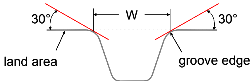
Figure A.1: Groove edge radius
